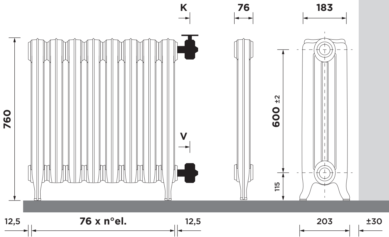
on the floor | bodenstehend | vloerstaand | на зemi | на полу/ногах AD760-F, all dimensions in mm ±2
