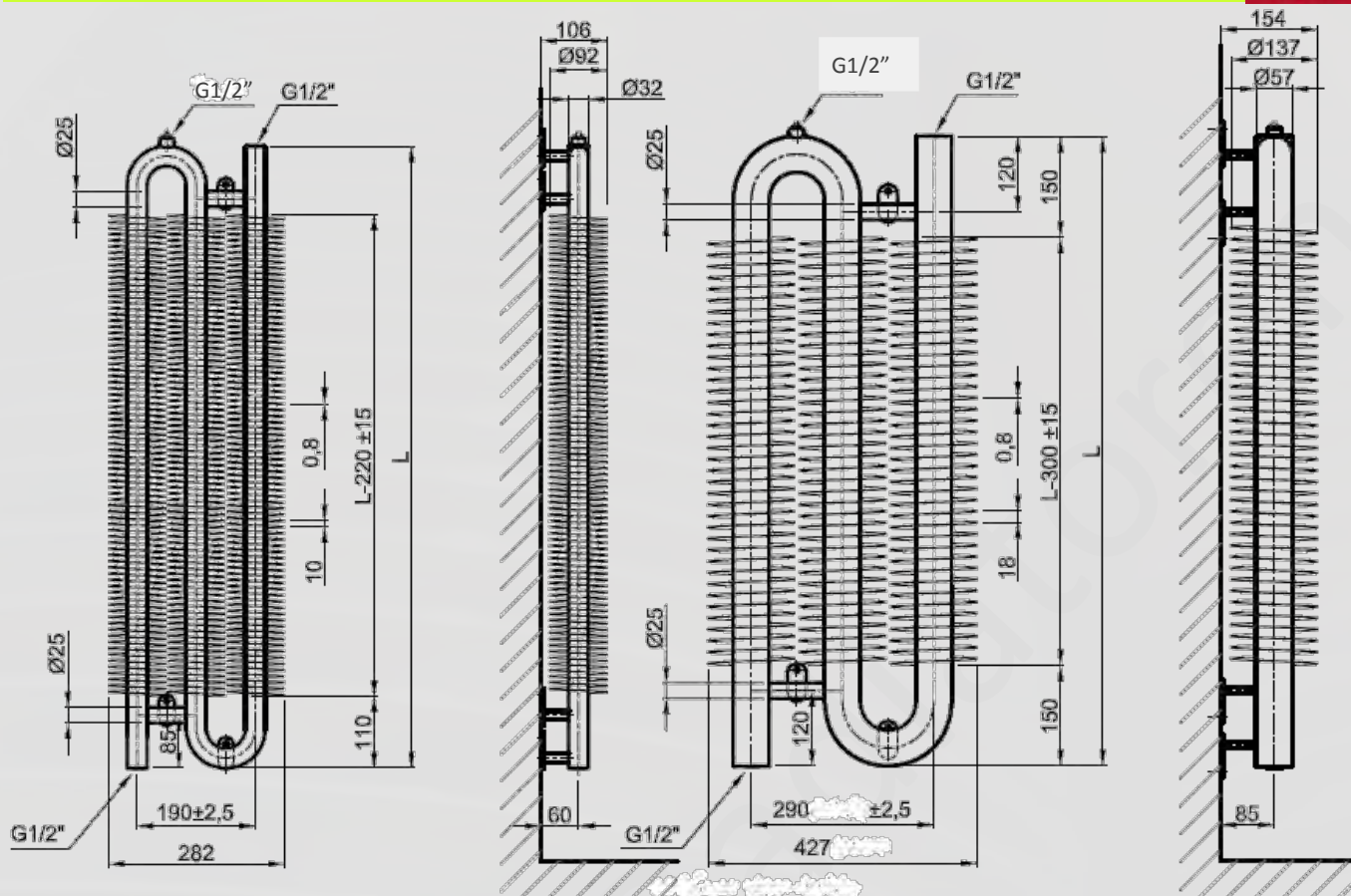
RA03 32×2×92 VERTICAL LEFT
